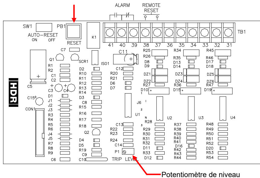
Figure 5.1 Carte de limitation / déclenchement de courant
