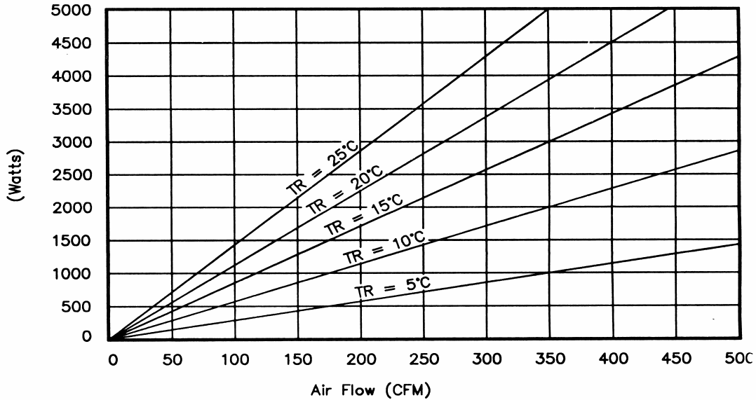
CHART 1 - Fan Requirements
